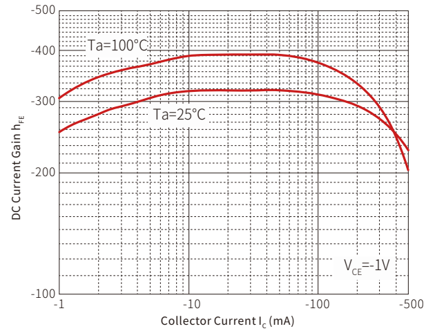
h_{FE} — I_C
