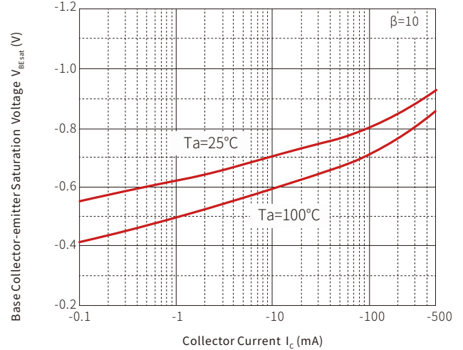
V_{BE\text{sat}} — I_C
