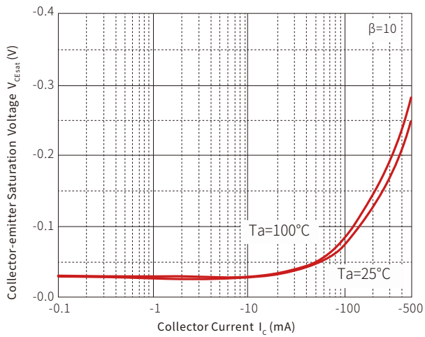
V_{CE\text{sat}} — I_C
