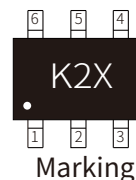
SOT-363
