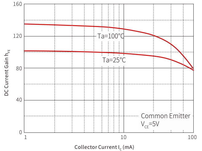
h_{FE} — I_C
