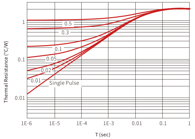
Fig. 4-Transient Thermal Impedance
